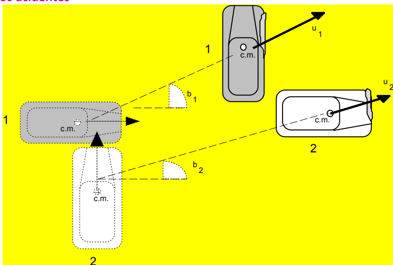
Figura 6 – Colisão perpendicular entre carros
